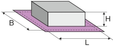
Formningsforholdet H:B for en kvadratisk form
