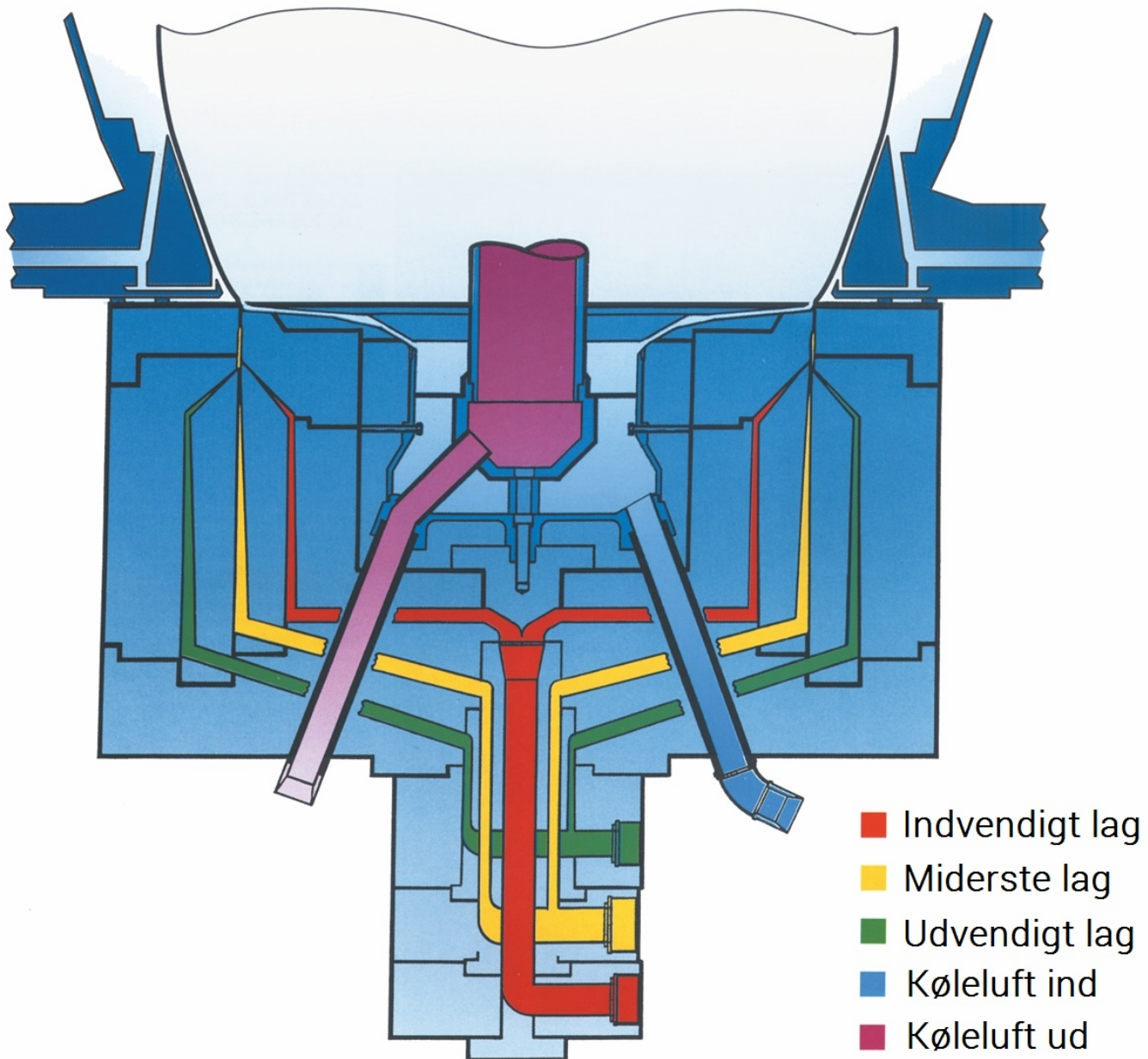
Tre-lags coekstruderingshoved med indvendig og udvendig køling
