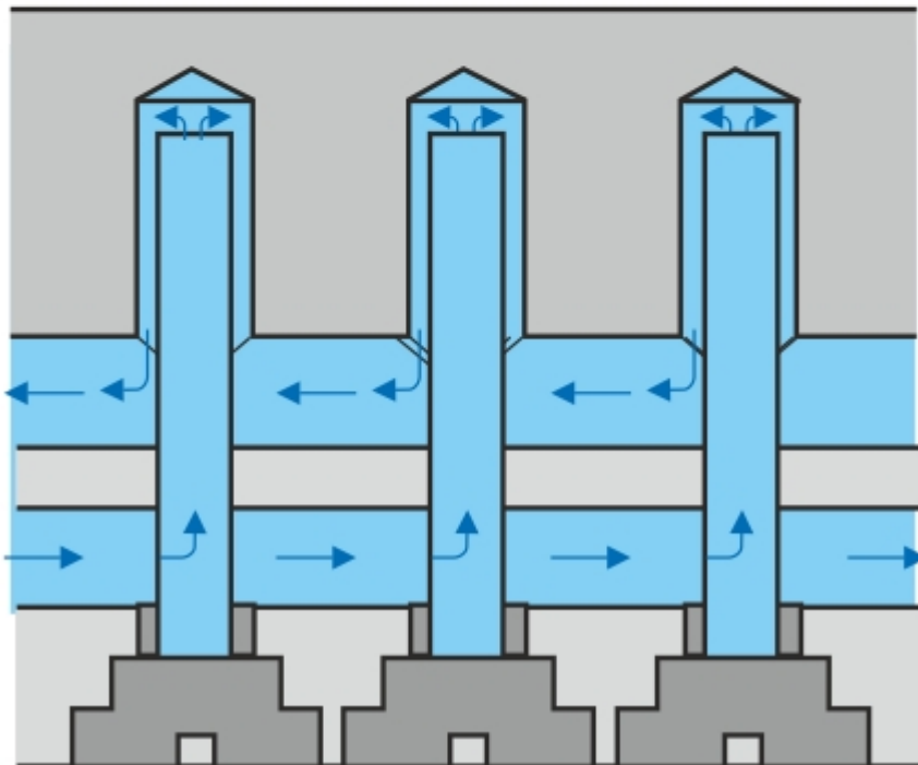
Gennemgående labyrintkøling
