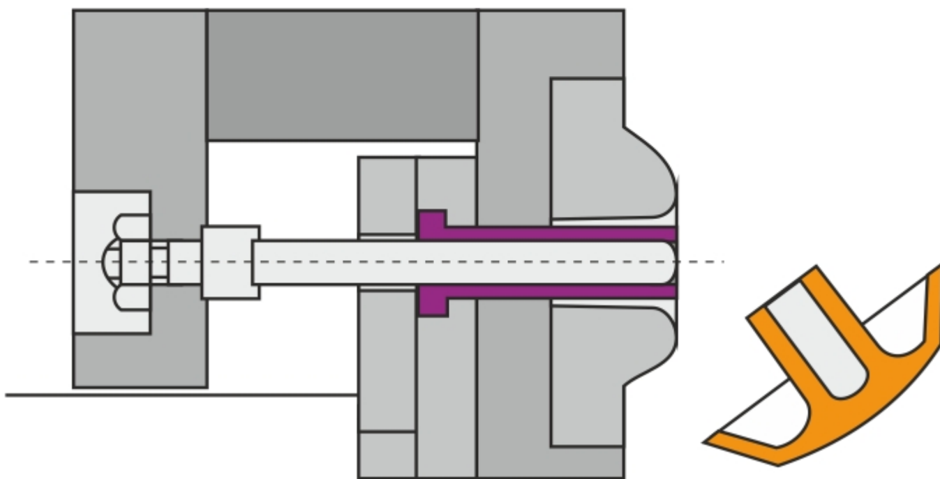
Almindelig rørstøderkonstruktion
