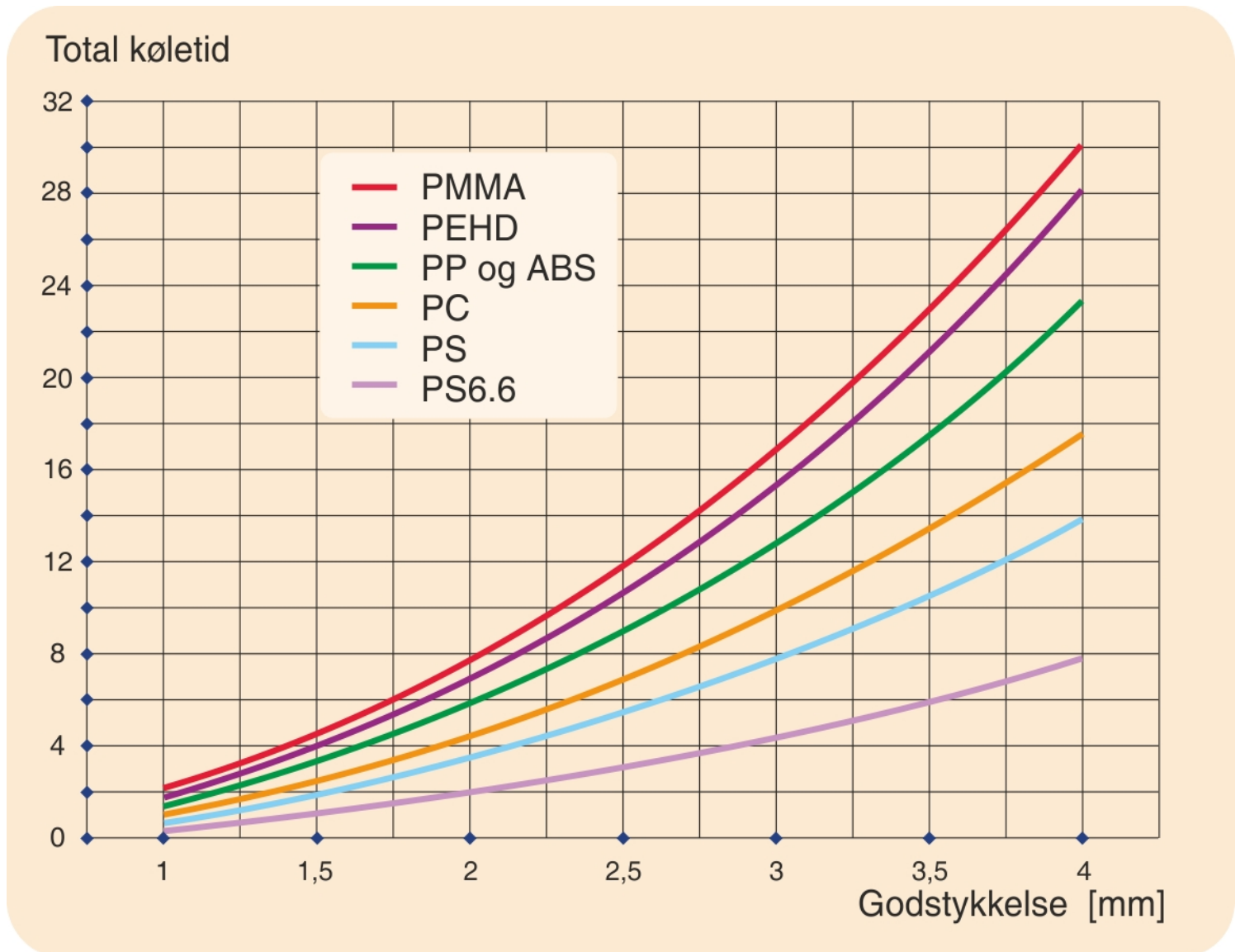
Køletidsdiagram
